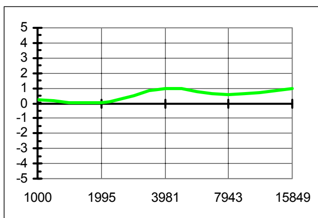
Influencia del TK-1000 sobre la respuesta del micrófono
