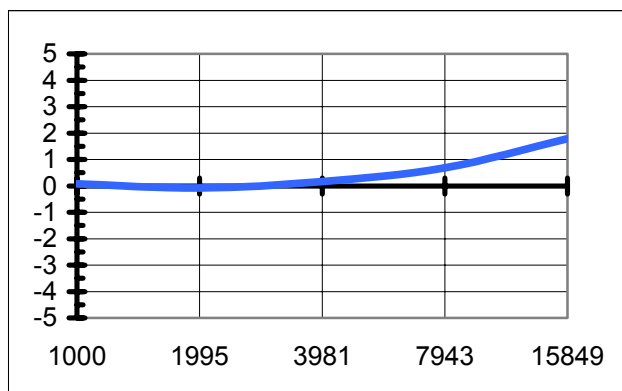
Influencia de la cubierta antilluvia sobre el micrófono
